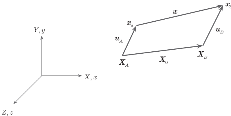
Figura 1: Movimento do elemento bi-articulado 3D.
