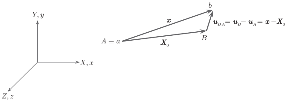
Figura 2: Vetor de deslocamentos nodais relativos.
