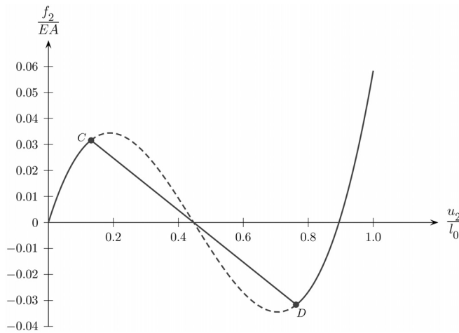
Figura 8: Trajetória secundária de equilíbrio.
