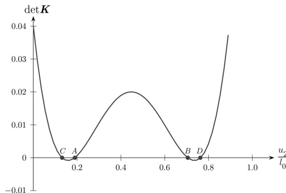
Figura 10: Determinante da matriz de rigidez tangente.
