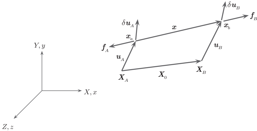
Figura 4: Vetor de forças nodais e a variação virtual dos deslocamentos nodais.
