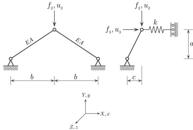
Figura 5: Trelça espacial com uma mola lateral.
