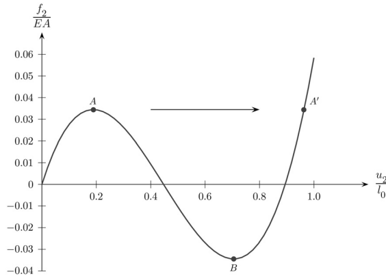
Figura 6: Trajetória primária de equilíbrio.
