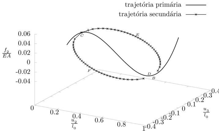
Figura 9: Trajetórias de equilíbrio em 3D.
