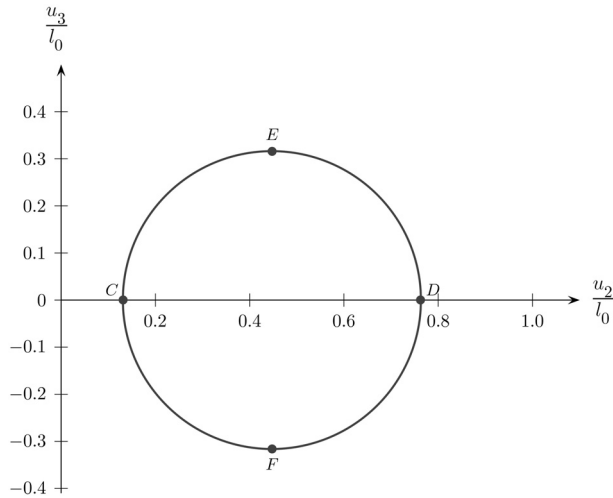
Figura 7: Curva no espaço de deslocamentos adimensionais.
