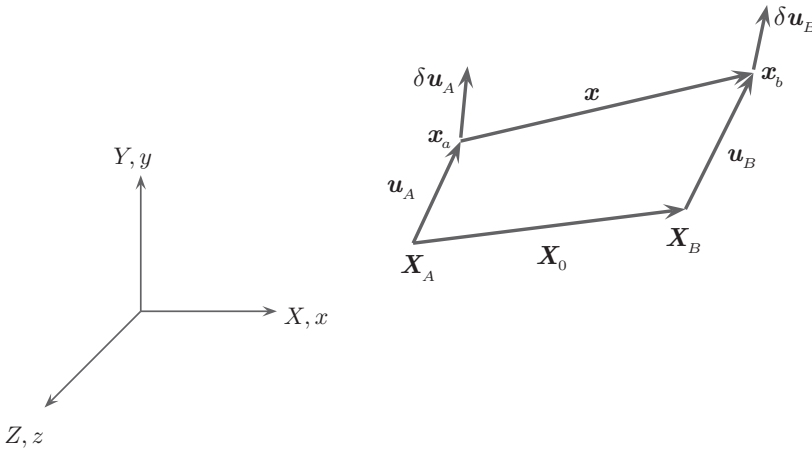
Figura 3: Variação virtual dos deslocamentos nodais.
