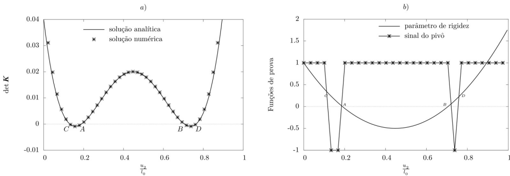
Figura 12: a) Determinante da matriz de rigidez tangente. b) Funções de prova.
