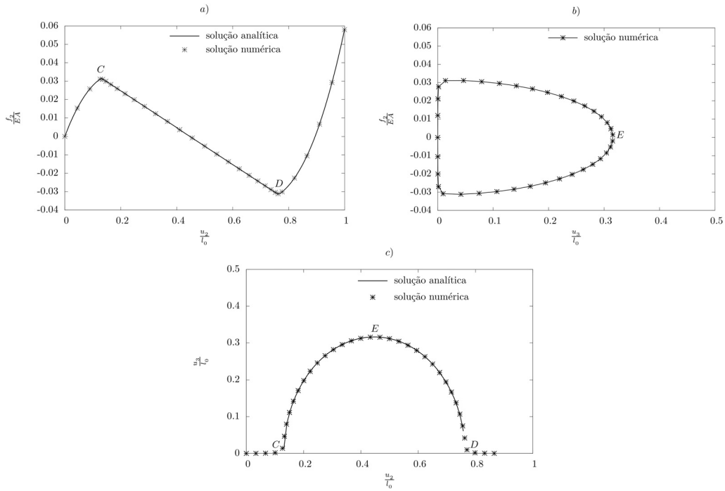
Figura 11: Trajetórias secundárias de equilíbrio. a) \mu_2 \times \lambda_2 . b) \mu_3 \times \lambda_2 . c) \mu_2 \times \mu_3 .
